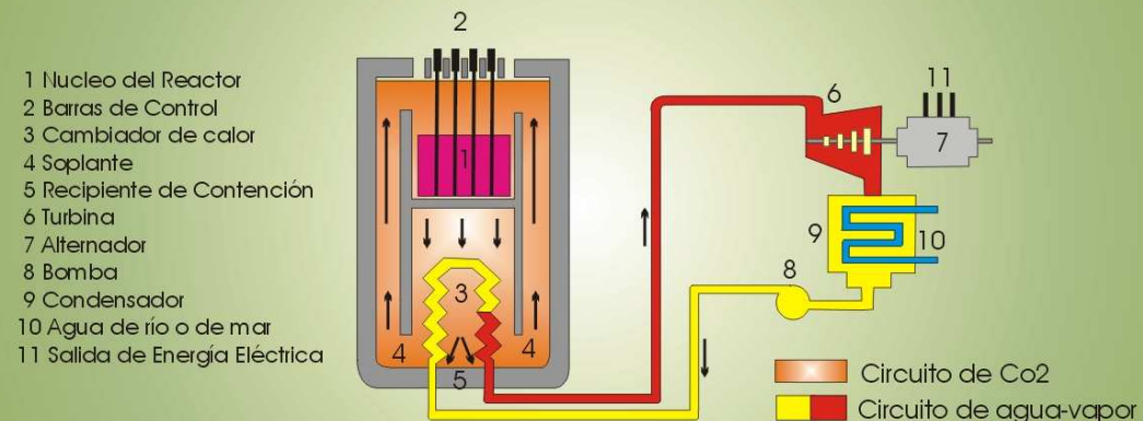
Esquema de una Central Nuclear con reactor de uranio natural
